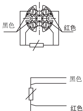
1 x Pt100, 4线式
