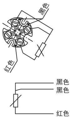
1 x Pt100, 3线式
