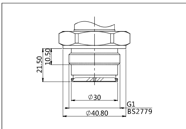
过程连接 (G03) (单位 : mm)
