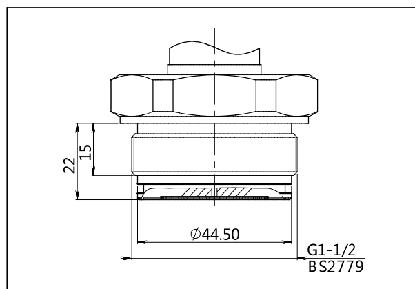
过程连接 (G07) (单位 : mm)
