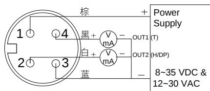
M12快速连接座
