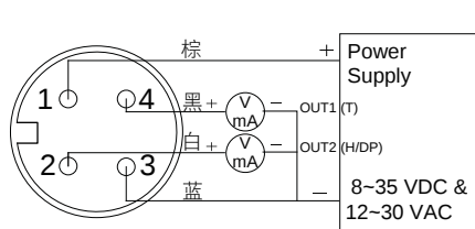
M12快速连接座
